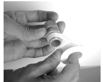
Figure 21 : Pose du joint téflon sur le porte-sonde.
